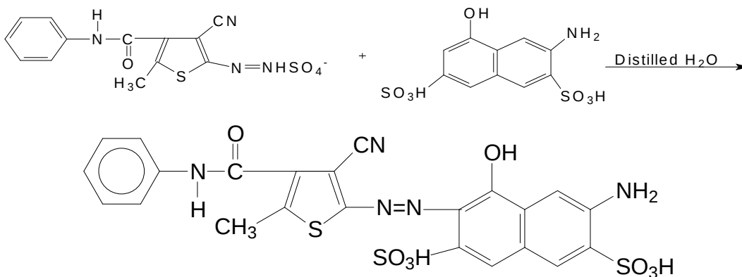
Dye 1a
